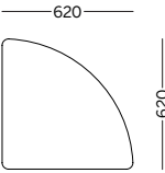
MODULE T3 - ¼ circle table top
