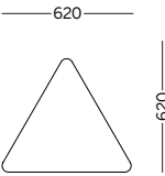
MODULE T4 - Triangular table top
